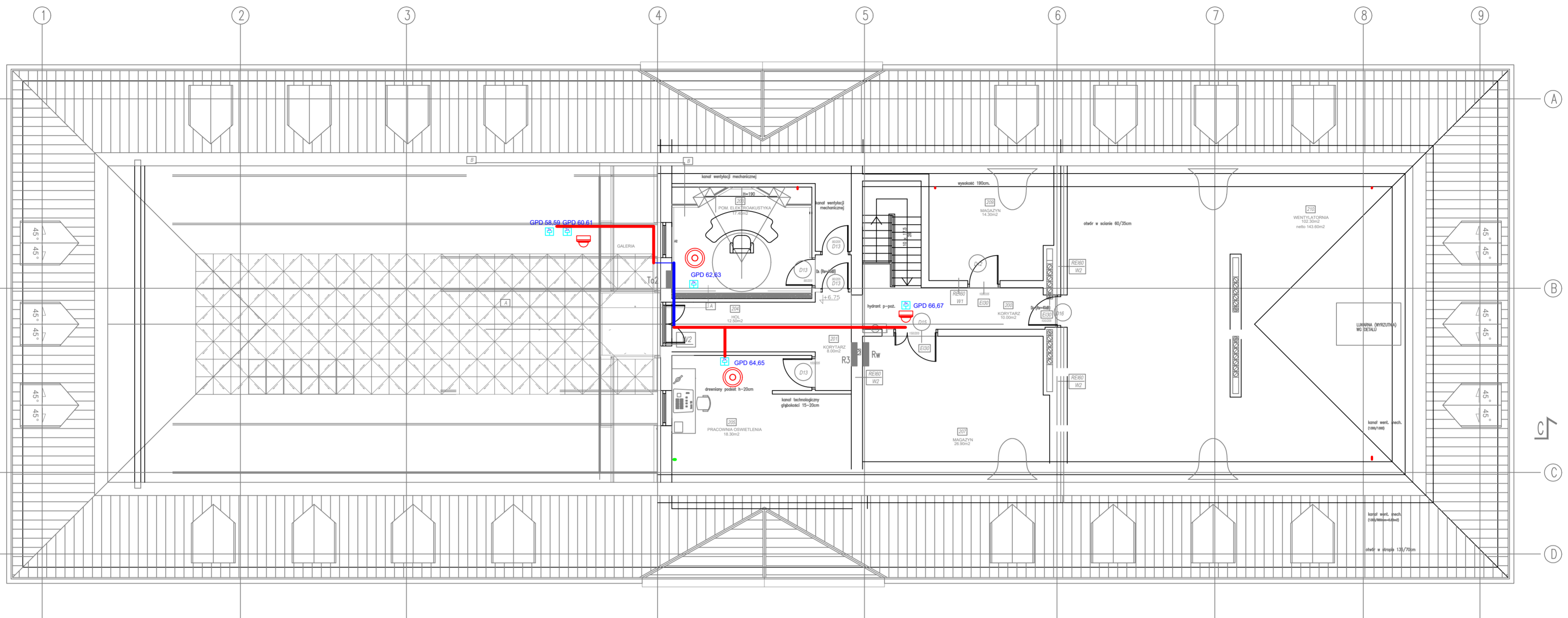
BUDYNEK GOSPODARCZY, poddasze, skala 1:100
