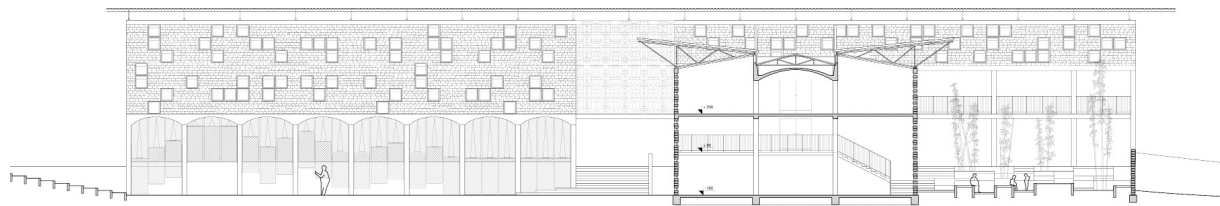
elevacja sali spotkań oraz przekrój przez część warsztatową
